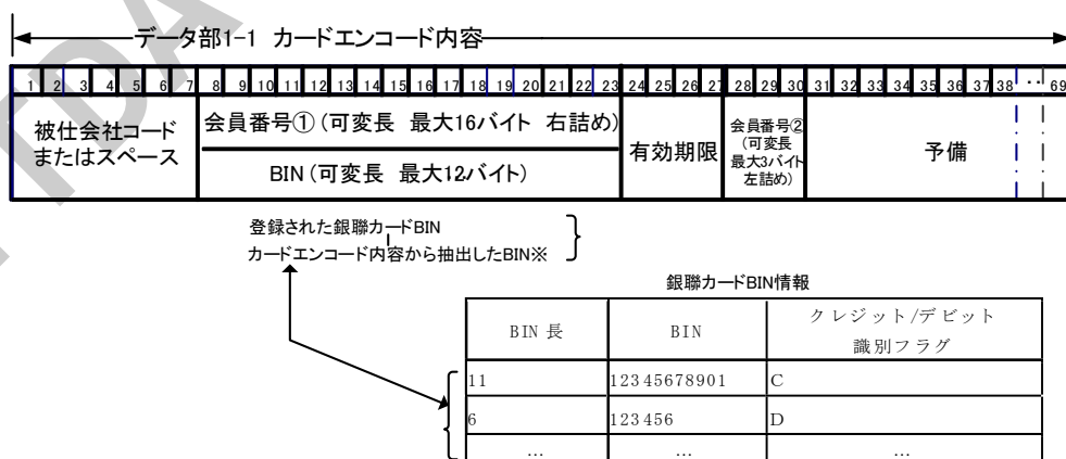
図 2-9 対象カード判定 (マニュアル入力時)
